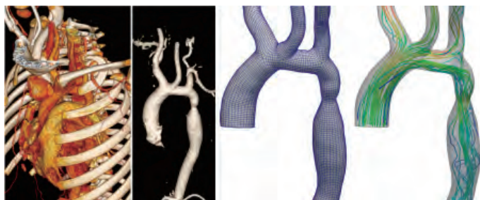
ヒト大動脈内の血流シミュレーション
